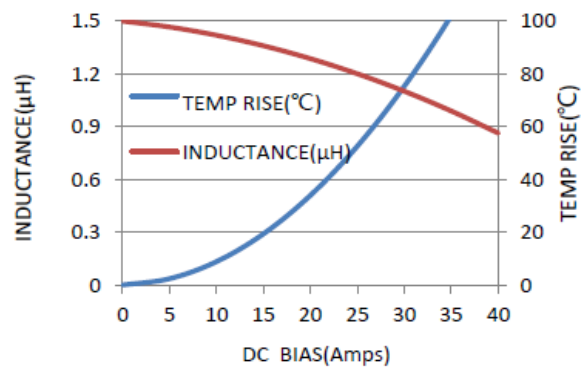
MCMB-1340-1R5MT
