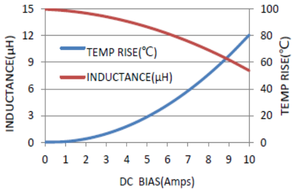
MCMB-1340-150MT
