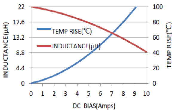
MCMB-1340-220MT
